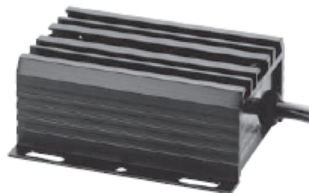
DC/DCコンバータ DC24VIN DC13.8V(5A)OUT DC24N-5C
