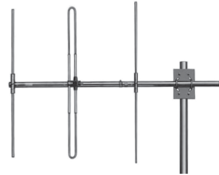
3素子八木アンテナ 3DV-450絶対利得8.15dB F/B比13dB
