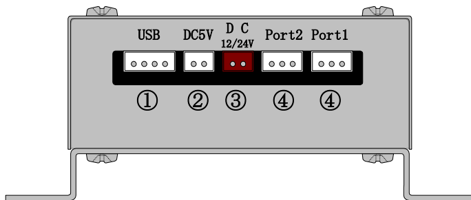
電源/IFケーブル接続部
